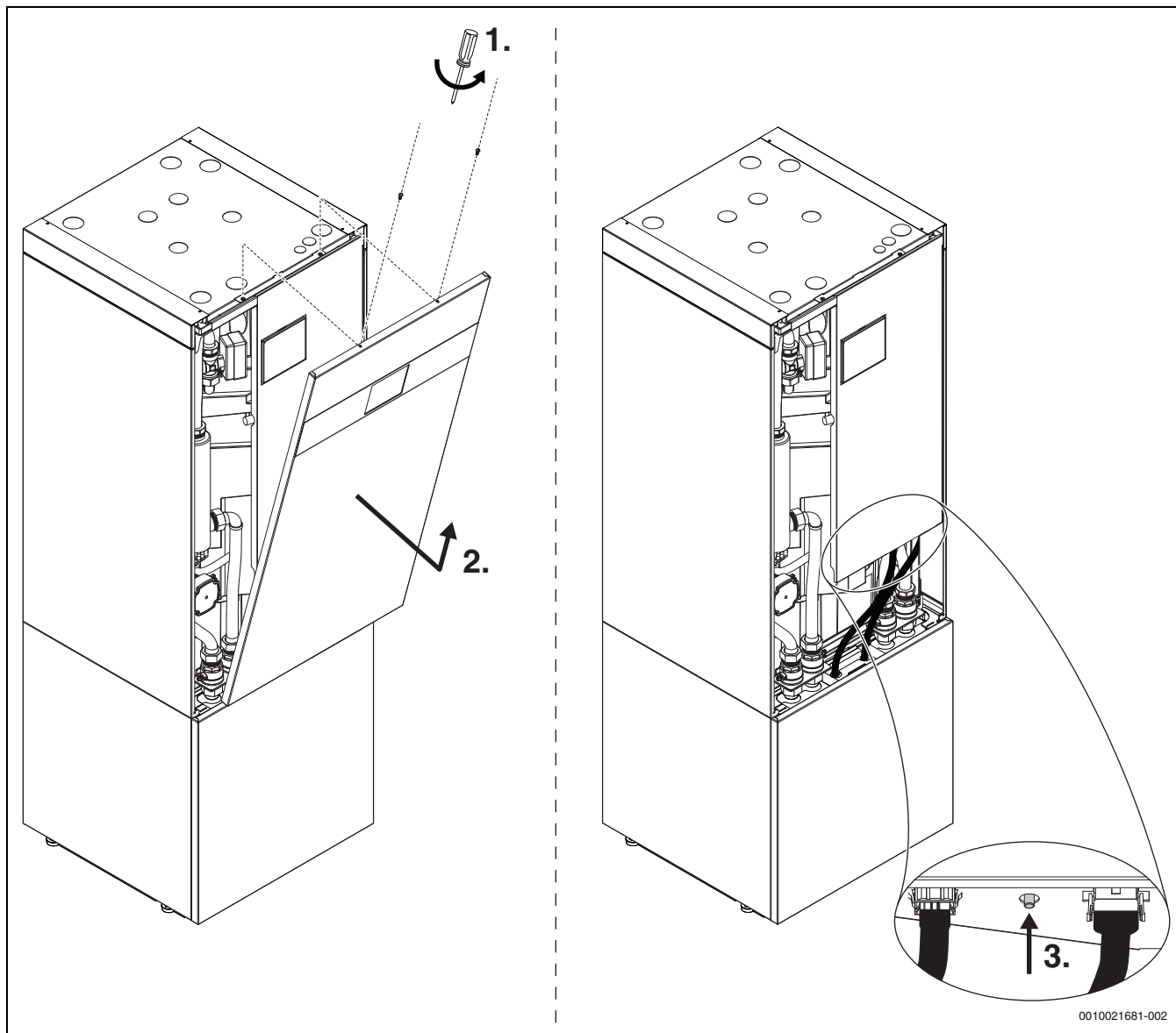
Bild 16 Återställning överhettningsskydd
